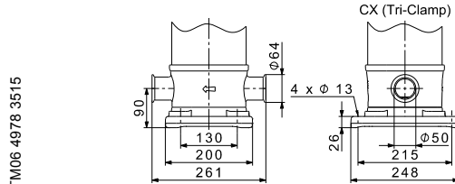
CRN-SF высоконапорный насос
