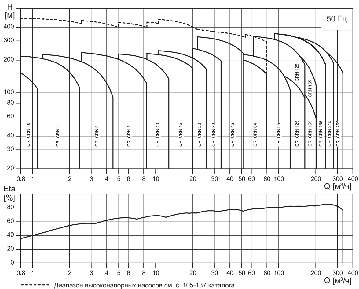
Рис. 3 Диапазон характеристик насосов CR, CRN 50 Гц
