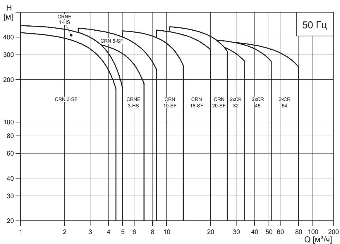
Рис. 19 Диапазон характеристик
