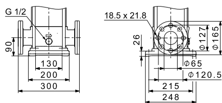
CRN питающий насос
